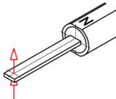
Transversale Zungensonde (PM2-TR, PM4-TR)
