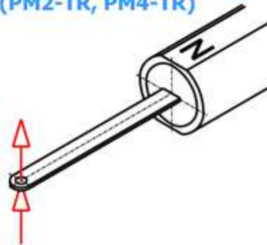
Transversale Zungensonde (PM2-TR, PM4-TR)
